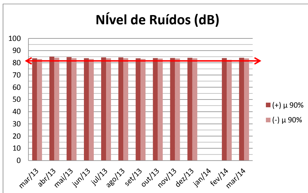
Gráfico 3-15 CCR Barcas – Nível de Ruído
